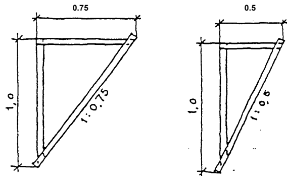
Mynd 6 Hallamæling.
